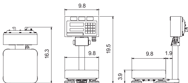
FS-6KiF / FS-15KiF
