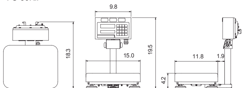
FS-30KiF
